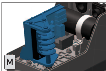
Mechanischer Endschalter
