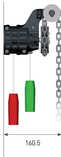
Manovra a catena Hand chain override Commande de secours à chaîne Maniobra manual con cadena
